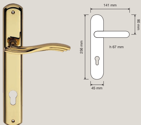
755 PL Maniglia con placca art.750 / Door handle on plate art.750
