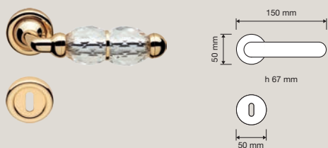
830 RB 103 Maniglia con rosetta art.103 / Door handle on rose art.103
