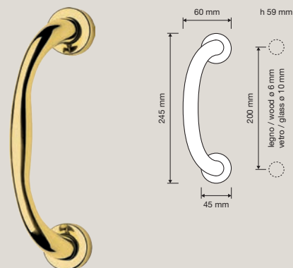
670 MN 200 101 Maniglione con rosette art.101 / Pull handle on roses art.101
