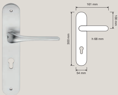
1454 PL Maniglia con placca art.1595 / Door handle on plate art.1595
