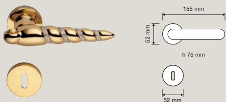
694 RB 023 Maniglia con rosetta art.023 / Door handle on rose art.023
