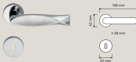
692 RB 023 Maniglia con rosetta art.023 / Door handle on rose art.023
