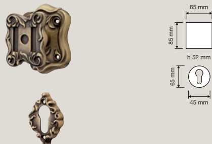
1308 PG 092 Pomolo a girare con rosetta art.092 / Turnable knob on rose art.092
