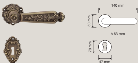
1210 RB 078 Maniglia con rosetta art.078 / Door handle on rose art.078
