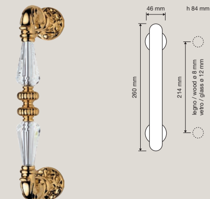
1542 MN 214 Maniglione. Attenzione: l'interasse può variare leggermente, chiedere sempre le misure prima di forare la porta. / Pull handle. Attention: the distance can have little changes, please always ask before making the holes in the door.
