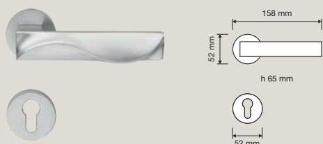
1410 RB 023 Maniglia con rosetta art.023 / Door handle on rose art.023
