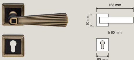
1055 RB 114 Maniglia con rosetta art.114 / Door handle on rose art.114
