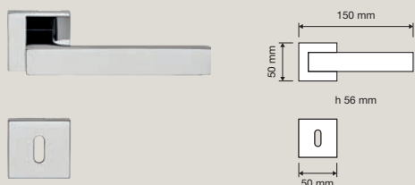
1156 RB 024 Maniglia con rosetta art.024 / Door handle on rose art.024
