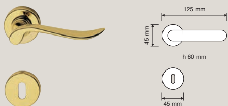
545 RB 101 Maniglia con rosetta art.101 / Door handle on rose art.101
