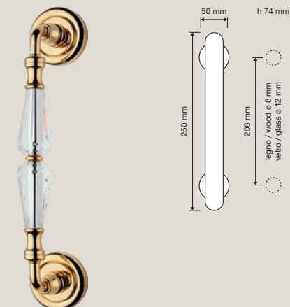
900 MN 208 103 Maniglione con rosette art.103. Attenzione: l'interasse può variare leggermente, chiedere sempre le misure prima di forare la porta. / Pull handle on roses art.103. Attention: the distance can have little changes, please always ask before making the holes in the door.
