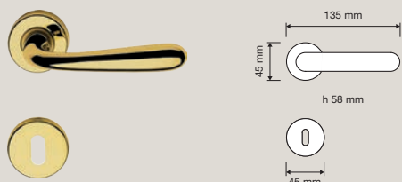
670 RB 101 Maniglia con rosetta art.101 / Door handle on rose art.101
