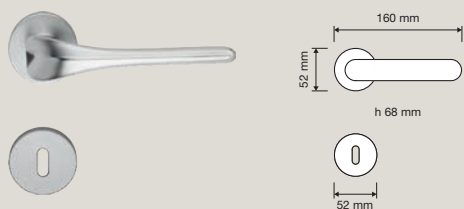
1450 RB 023 Maniglia con rosetta art.023 / Door handle on rose art.023
