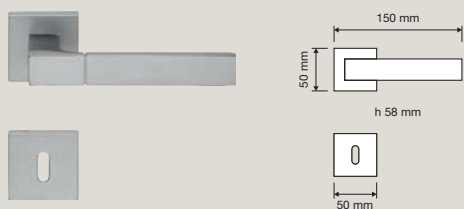
1155 RB 019 Maniglia con rosetta art.019 / Door handle on rose art.019
