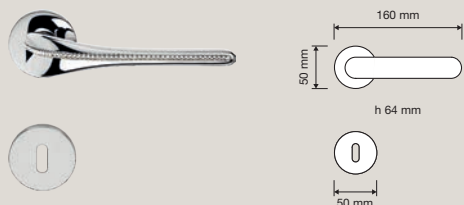
1451 RB 025 Maniglia con rosetta art.025 / Door handle on rose art.025
