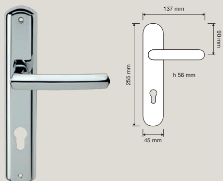
509 PL Maniglia con placca / Door handle on plate
