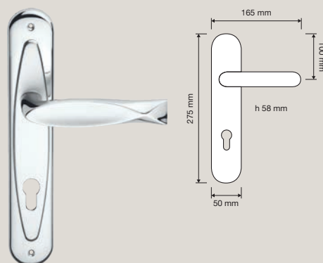
692 PL Maniglia con placca art.955 / Door handle on plate art.955
