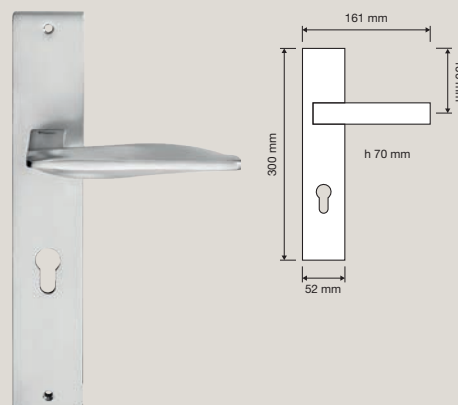
1440 PL Maniglia con placca / Door handle on plate
