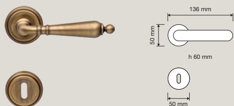
1460 RB 011 Maniglia con rosetta art.011 / Door handle on rose art.011
