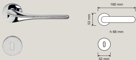
1451 RB 023 Maniglia con rosetta art.023 / Door handle on rose art.023
