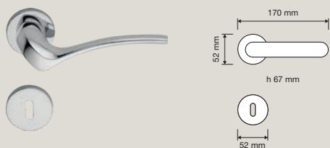
691 RB 023 Maniglia con rosetta art.023 / Door handle on rose art.023
