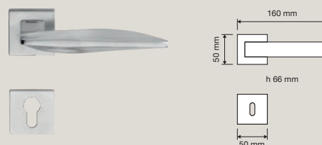
1440 RB 024 Maniglia con rosetta art.024 / Door handle on rose art.024
