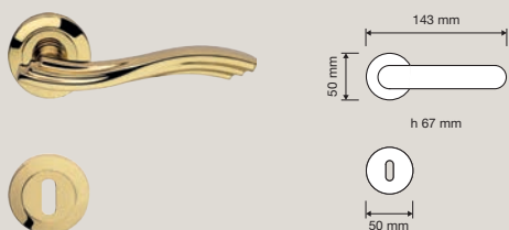
755 RB 102 Maniglia con rosetta art.102 / Door handle on rose art.102
