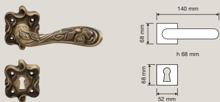
1165 RB 091 Maniglia con rosetta art.091 / Door handle on rose art.091
