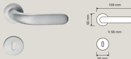
1595 RB 025 Maniglia con rosetta art.025 / Door handle on rose art.025
