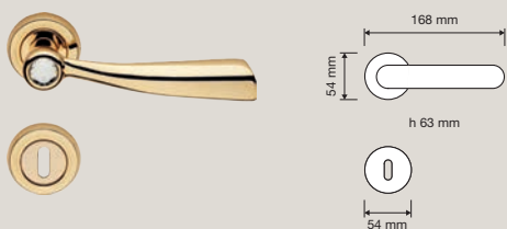
991 RB 108 Maniglia con rosetta art.108 / Door handle on rose art.108
