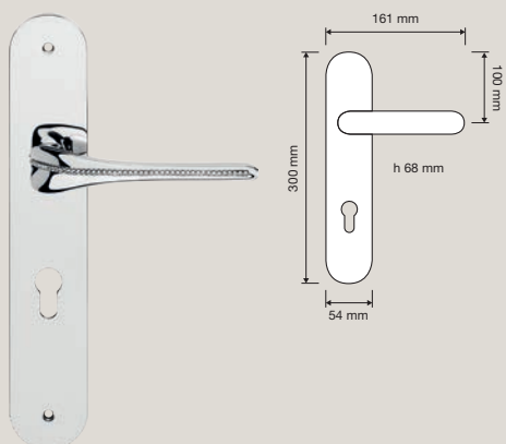
1453 PL Maniglia con placca art.1595 / Door handle on plate art.1595
