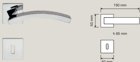
1041 RB 024 Maniglia con rosetta art.024 / Door handle on rose art.024
