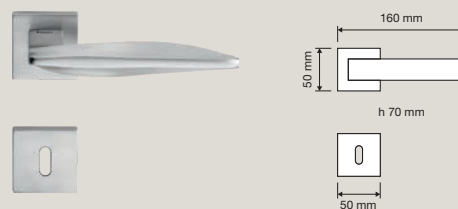
1440 RB 019 Maniglia con rosetta art.019 / Door handle on rose art.019
