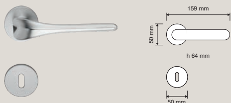
1450 RB 025 Maniglia con rosetta art.025 / Door handle on rose art.025
