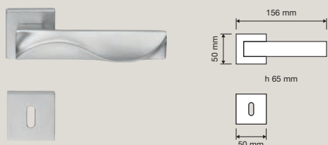
1410 RB 019 Maniglia con rosetta art.019 / Door handle on rose art.019
