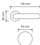
262 B4 Limitatore con rosetta art.101 / Limiting device on rose art.101
