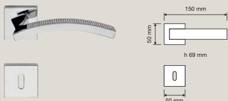
1041 RB 019 Maniglia con rosetta art.019 / Door handle on rose art.019
