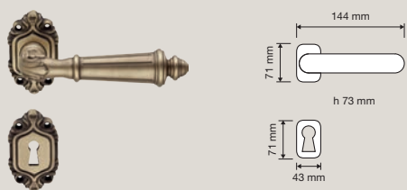
1610 RB 005 Maniglia con rosetta art.005 / Door handle on rose art.005
