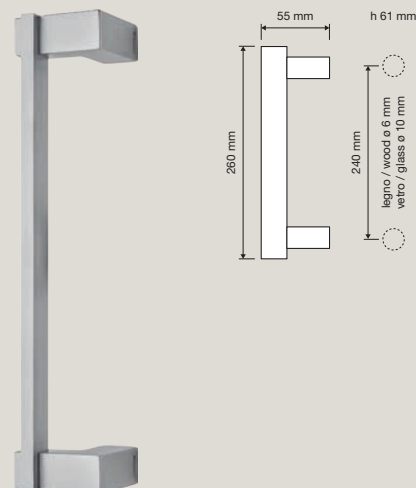
1110 MZ 240 Maniglione zancato. Interassi disponibili 240-300-400-600- 800. / Offset pull handle. Available distances 240-300- 400-600-800.
