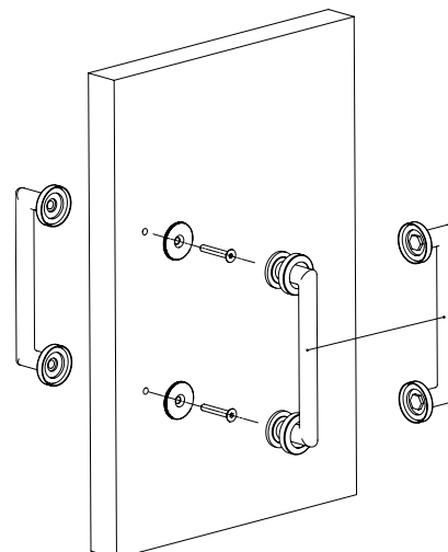
Montaggio coppia di maniglioni con rosetta 011-102-103 / Fitting of pull handle couple with rose 011-102-103
