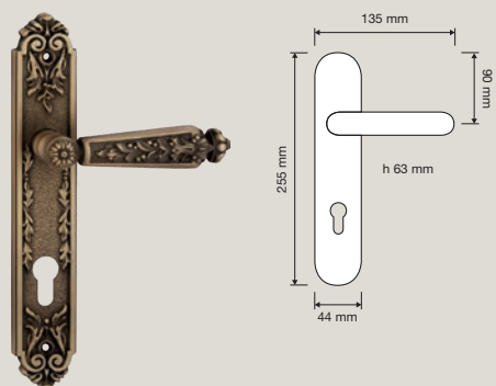
1210 PL Maniglia con placca / Door handle on plate
