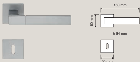
1155 RB 024 Maniglia con rosetta art.024 / Door handle on rose art.024
