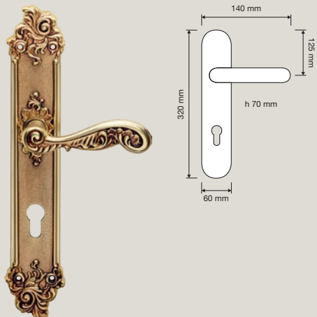
1285 PL Maniglia con placca / Door handle on plate
