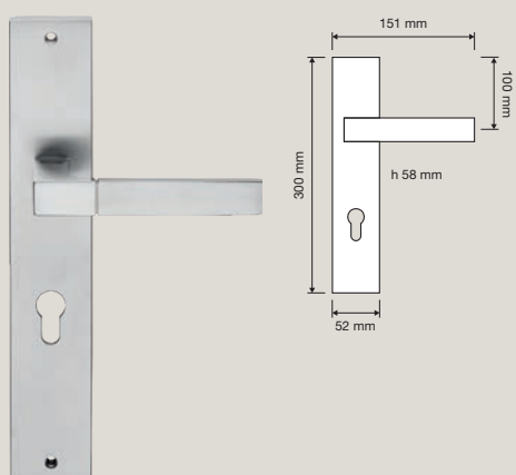
1150 PL Maniglia con placca art.1104 / Door handle on plate art.1104
