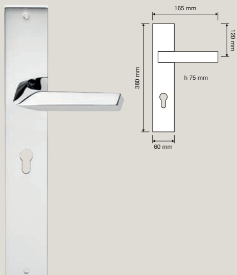
1421 PL Maniglia con placca art.1106 / Door handle on plate art.1106
