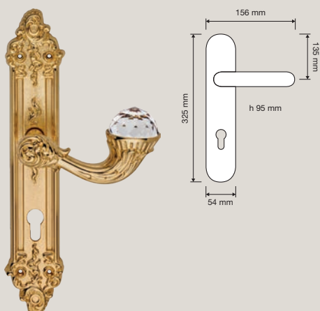
1526 PL Maniglia con placca art.1308 / Door handle on plate art.1308
