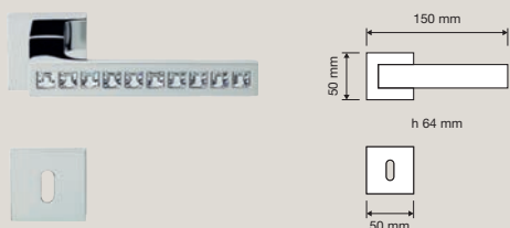
1215 RB 024 Maniglia con rosetta art.024 / Door handle on rose art.024
