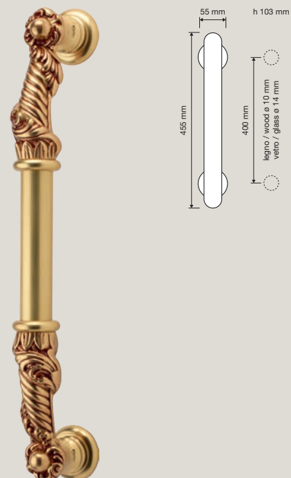
1285 MN 400 Maniglione. Interassi disponibili 400-500- 600. / Pull handle. Available distances 400-500-600.
