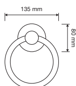
Leone 351 BA 110 Battente con anello / Door knocker with ring
