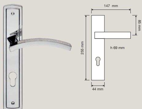
1041 PL Maniglia con placca art.1040 / Door handle on plate art.1040
