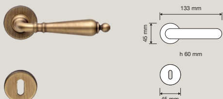
1460 RB 101 Maniglia con rosetta art.101 / Door handle on rose art.101
