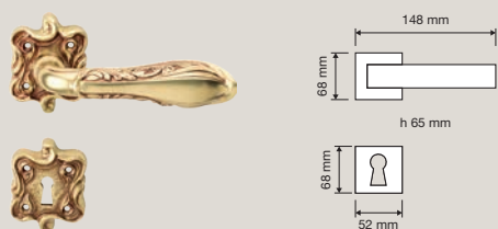
1160 RB 091 Maniglia con rosetta art.091 / Door handle on rose art.091
