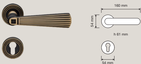
1055 RB 112 Maniglia con rosetta art.112 / Door handle on rose art.112
