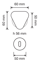
Open 1105 PG 019 Pomolo a girare con rosetta art.019 / Turnable knob on rose art.019
