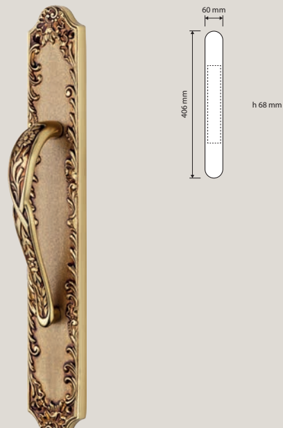
1395 SL Maniglione su placca / Pull handle on plate
