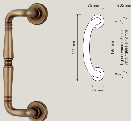
1460 MZ 198 101 Maniglione zancato con rosette art.101 / Offset Pull handle on roses art.101
