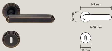
1670 RB 004 Maniglia con rosetta art.004 / Door handle on rose art.004
