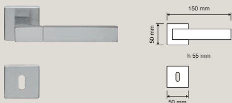
1155 RB 088 Maniglia con rosetta art.088 / Door handle on rose art.088
