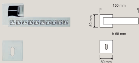
1215 RB 019 Maniglia con rosetta art.019 / Door handle on rose art.019
