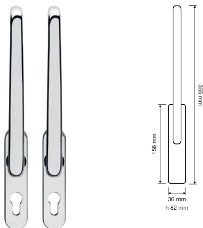
Komfort 1617 MC Maniglione alzante accoppiato foro yale / Set pull handles cylinder hole
