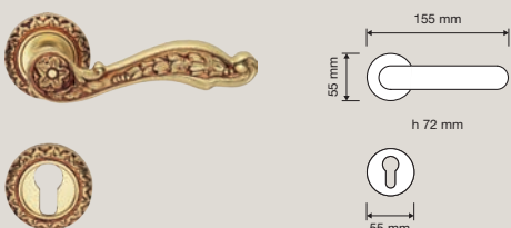
1560 RB 115 Maniglia con rosetta art.115 / Door handle on rose art.115
