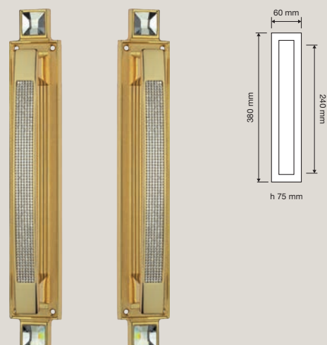
1056 AP Maniglione accoppiato su placca / Set pull handles on plate
