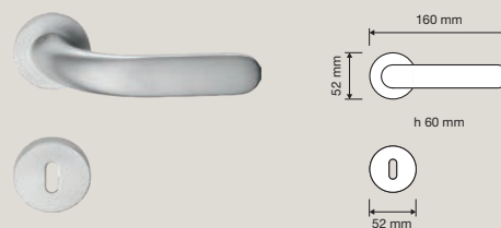
1595 RB 023 Maniglia con rosetta art.023 / Door handle on rose art.023
