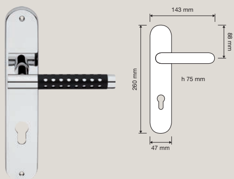
1726 PL Maniglia con placca art.123 / Door handle on plate art.123
