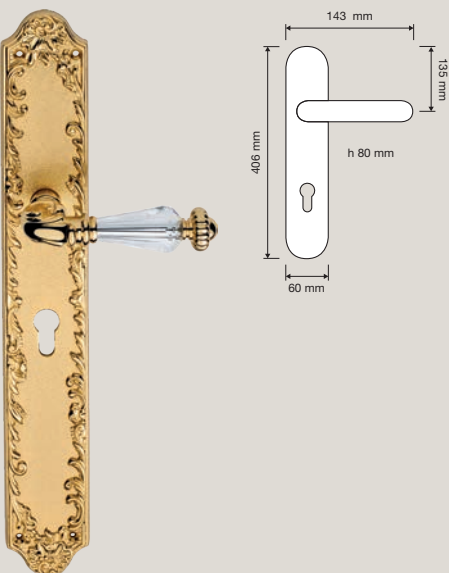
1542 PL Maniglia con placca art.1395 / Door handle on plate art.1395
