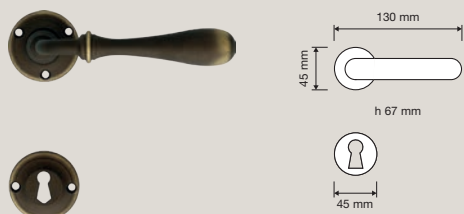
745 RB 110 Maniglia con rosetta art.110 / Door handle on rose art.110
