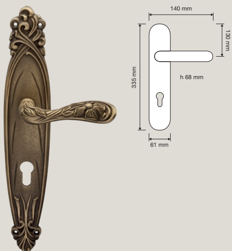
1165 PL Maniglia con placca / Door handle on plate
