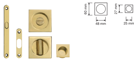
184 KT Kit incasso quadrato con nottolino, taglio cacciavite, maniglia trascinamento e serratura / Square inset handle kit with thumb, finger pull and locking system
