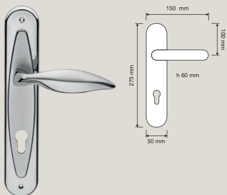
955 PL Maniglia con placca / Door handle on plate
