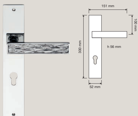
1645 PL Maniglia con placca / Door handle on plate
