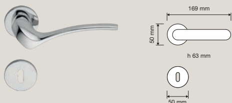
691 RB 025 Maniglia con rosetta art.025 / Door handle on rose art.025
