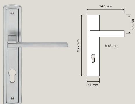
1110 PL Maniglia con placca / Door handle on plate
