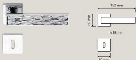
1645 RB 019 Maniglia con rosetta art.019 / Door handle on rose art.019
