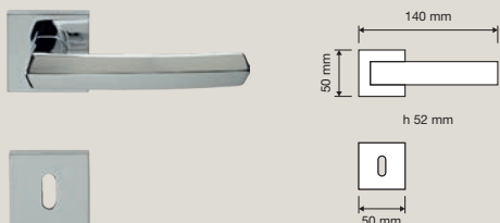
509 RB 024 Maniglia con rosetta art.024 / Door handle on rose art.024
