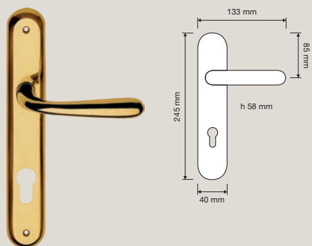
670 PL Maniglia con placca / Door handle on plate
