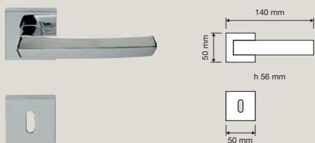
509 RB 019 Maniglia con rosetta art.019 / Door handle on rose art.019
