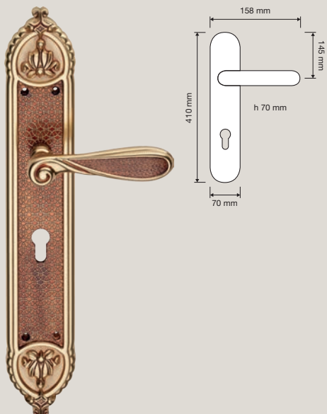
1651 PL Maniglia con placca Big / Door handle on plate Big
