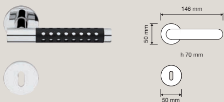
1726 RB 025 Maniglia con rosetta art.025 / Door handle on rose art.025
