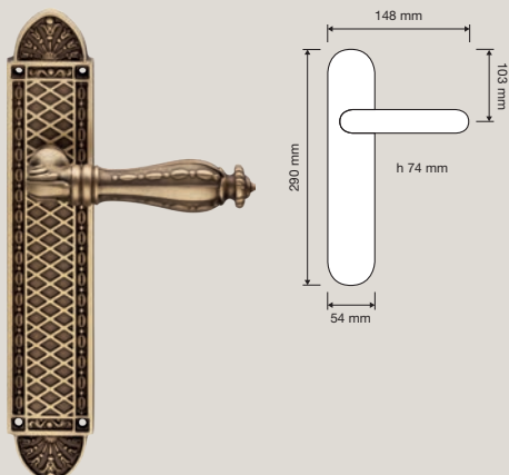
1563 PL Maniglia con placca Small art.1563 / Door handle on plate Small art.1563
