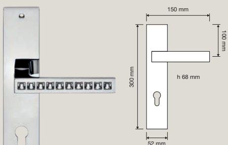
1216 PL Maniglia con placca art.1104 / Door handle on plate art.1104
