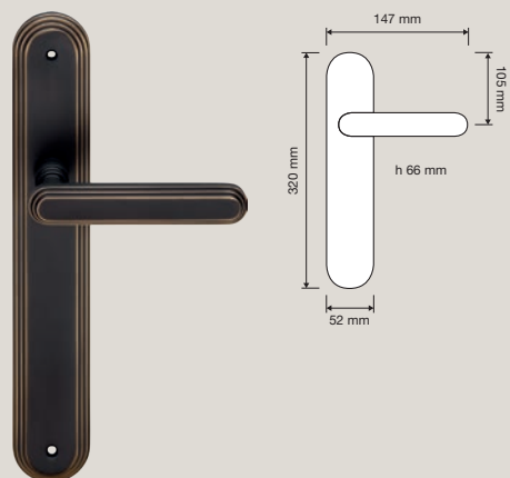
1670 PL Maniglia con placca / Door handle on plate
