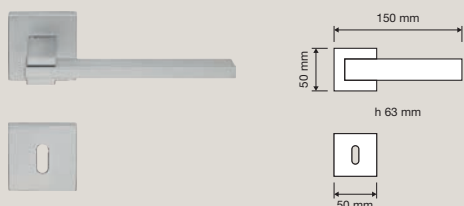
1110 RB 019 Maniglia con rosetta art.019 / Door handle on rose art.019
