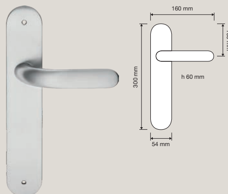
1595 PL Maniglia con placca / Door handle on plate
