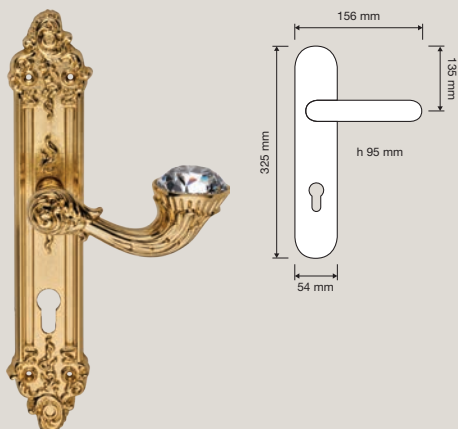
1527 PL Maniglia con placca art.1308 / Door handle on plate art.1308
