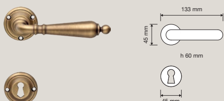
1460 RB 110 Maniglia con rosetta art.110 / Door handle on rose art.110
