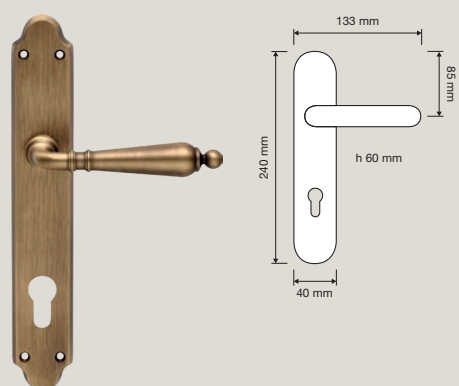
1460 PL Maniglia con placca / Door handle on plate
