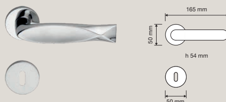
692 RB 025 Maniglia con rosetta art.025 / Door handle on rose art.025
