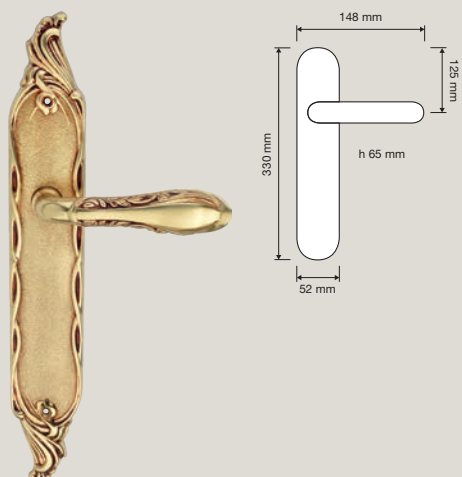
1160 PL Maniglia con placca / Door handle on plate
