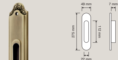
1390 IP Placca incasso su placca / Flush pull on plate
