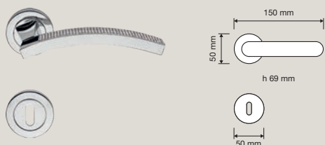
1041 RB 102 Maniglia con rosetta art.102 / Door handle on rose art.102
