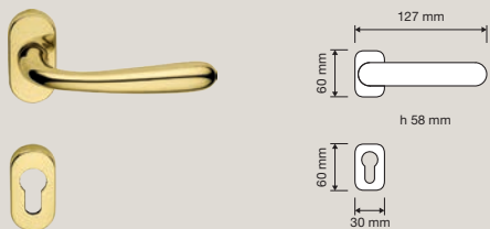
670 RB 096 Maniglia con rosetta art.096 / Door handle on rose art.096
