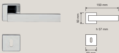
1156 RB 088 Maniglia con rosetta art.088 / Door handle on rose art.088
